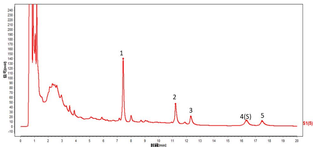
对照特征图谱 峰 4 (S)：异茜草素 色谱柱：CORTECS T3 (2.1mm×100mm, 1.6 \mu m)
