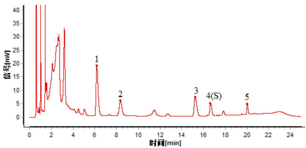
峰 1：腺嘌呤；峰 2：鸟苷；峰 4（S）：腺苷； 僵蚕配方颗粒对照特征图谱 色谱柱：Triart C18；2.1mm×100mm，1.9μm
