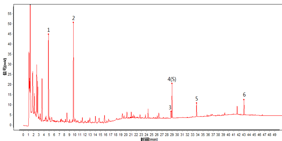
峰 3：黄豆黄素；峰 4（S）：大豆苷元；峰 5：染料木素 淡豆豉配方颗粒对照特征图谱 色谱柱：BEH Shield RP18；2.1mm×150mm，1.7μm
