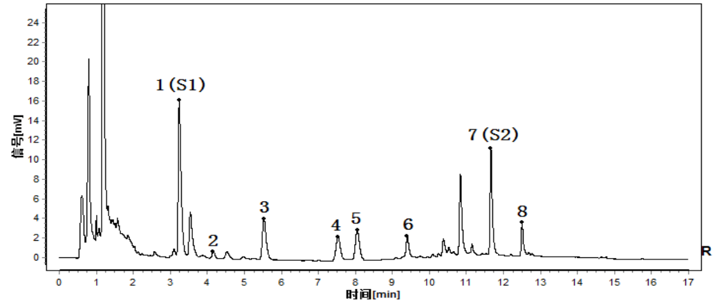
峰 1 (S1): 橙黄决明素; 峰 3: 黄决明素; 峰 6: 大黄素; 峰 7 (S2): 大黄酚; 峰 8: 大黄素甲醚 炒决明子 (钝叶决明) 配方颗粒对照特征图谱 色谱柱: Agilent SB C18 (2.1mm×100mm, 1.8μm)
