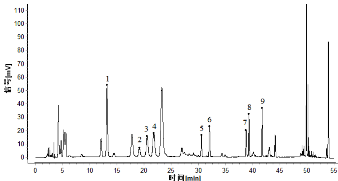
图 1 炒鸡内金配方颗粒对照特征图谱
