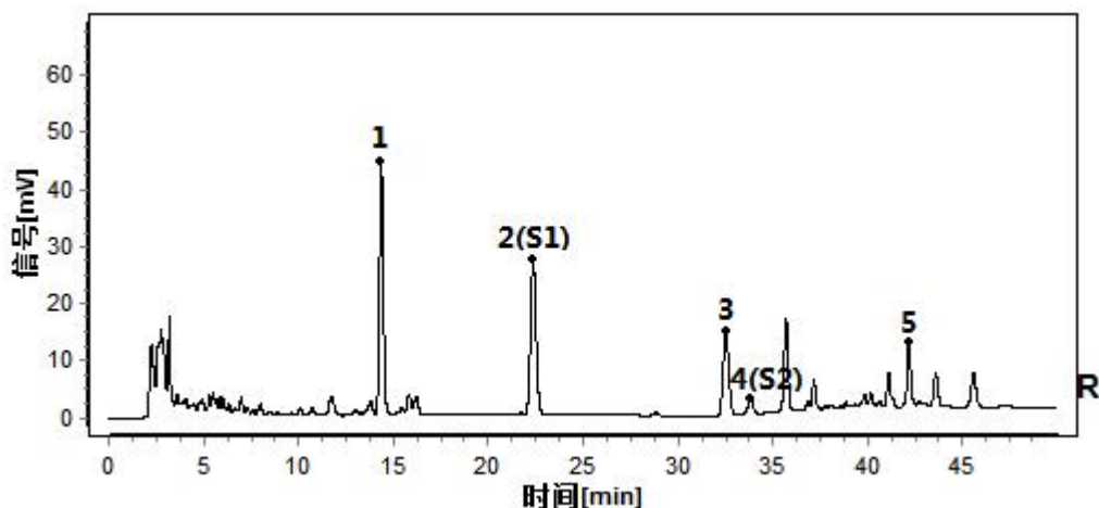
峰 2 (S1): 11-羰基- \beta -乙酰乳香酸; 峰 4 (S2): \alpha -乳香酸 图 乳香 (埃塞俄比亚乳香) 配方颗粒对照特征图谱 色谱柱: Xbridge C18 (250mm \times 4.6mm, 5 \mu m)
